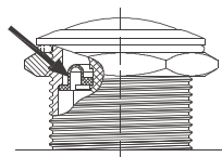
内置防水圈 Built-in waterproof ring
